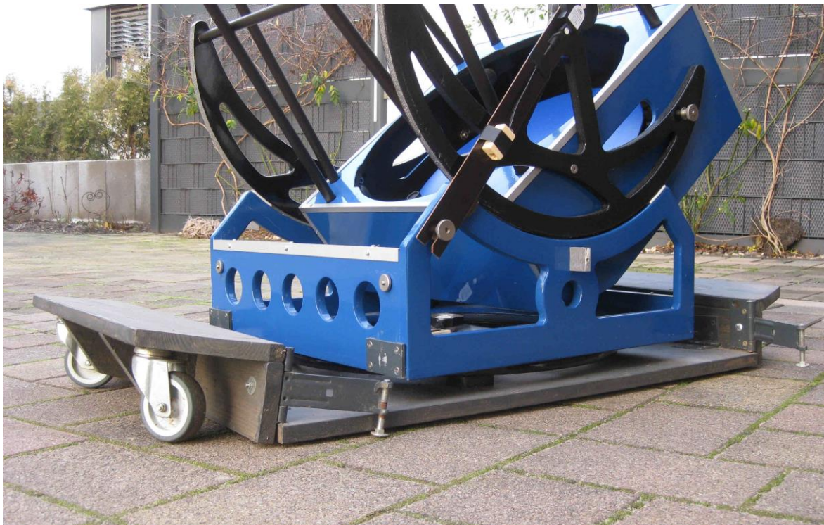
Ansicht der abgesenkten Plattform mit den hochgeklappten Rädern.
